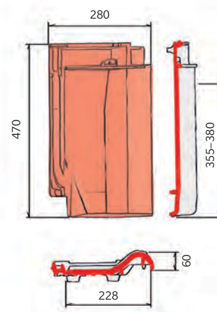
Rozměry základní tašky [mm]
