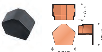
zamknięcie końcowe kalenicy nr 14
