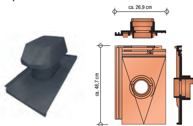
kominek odpowietrzający + czapa
