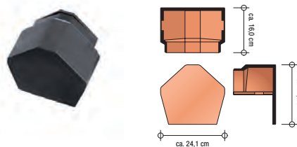
zamknięcie początkowe kalenicy
