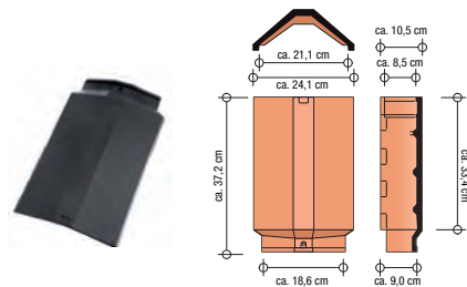
zamknięcie początkowe kalenicy
