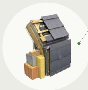
Rozwiązanie połączenia dachu i elewacji przy użyciu ukrytej rynny.
