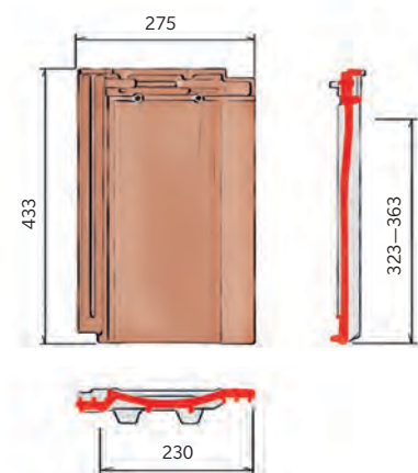
Rozměry základní tašky [mm]
