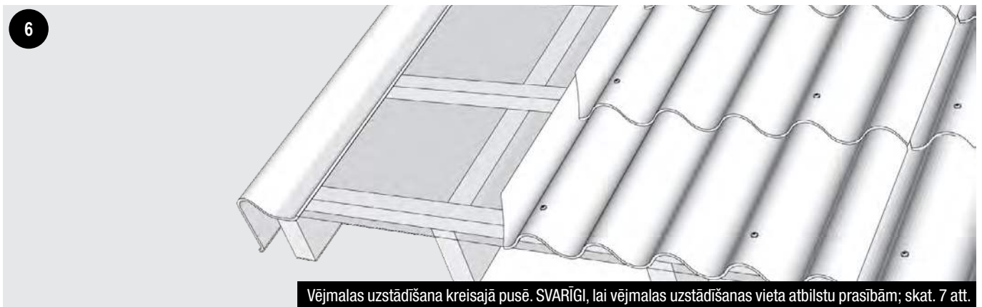
Otrās rindas pirmās viļņotās loksnes uzstādīšana. Viļņoto lokšņu pārļaidums ir 47 mm
